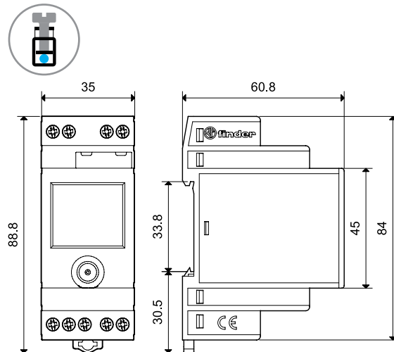
11.91 Schraubklemmen
